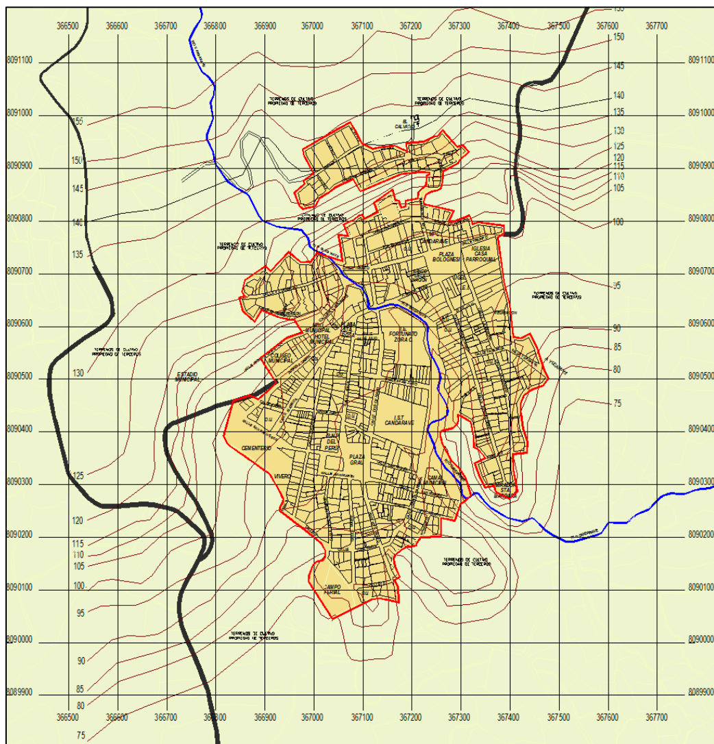
Figura N° 44: Topografía de la ciudad de Candarave curvas de nivel cada 5 m.
