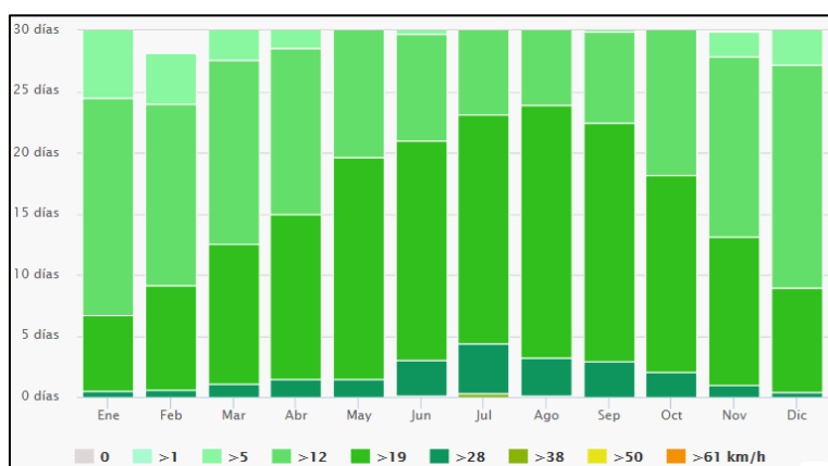
Figura N° 47: Velocidad promedio anual
