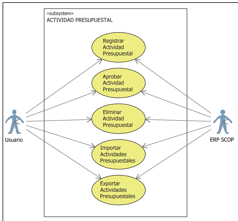
Figura 16. Diagrama de caso de uso Mantenimiento de Actividades Presupuestales
