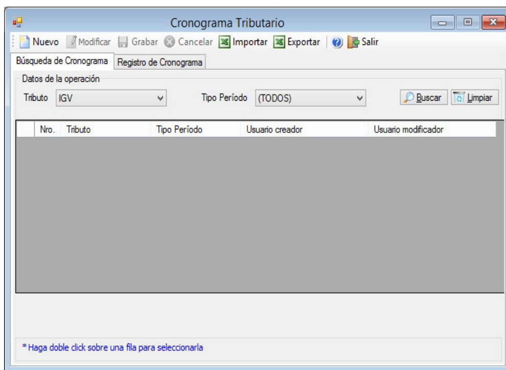
Figura 45. Mantenimiento del Cronograma Tributario SUNAT – pestaña de búsqueda
