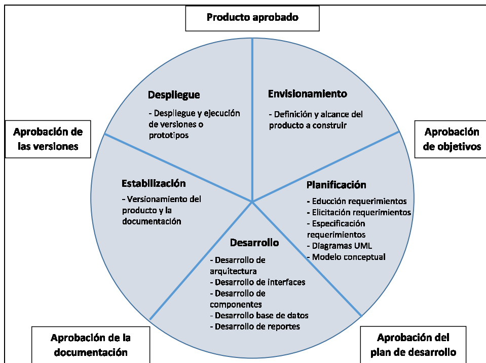
Figura 2. Tareas Proyecto Contabilidad vs MSF + Agile
