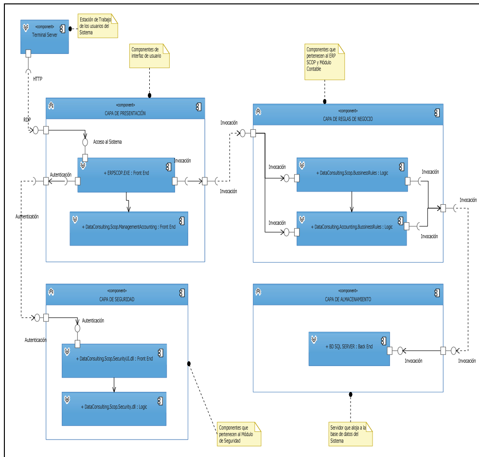
Arquitectura del SCOPCONTABLE
