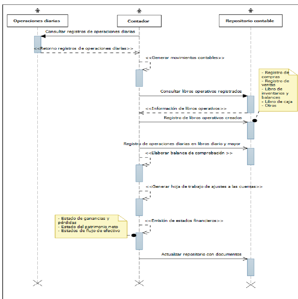
Figura 5. Diagrama de secuencia Contabilización Administrativa
