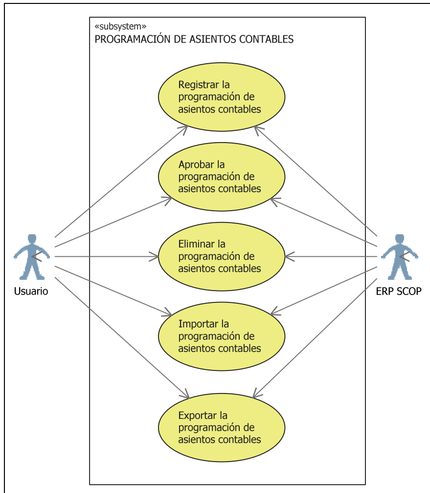
Figura 22. Diagrama de caso de uso Mantenimiento de las Programaciones de Asientos Contables
