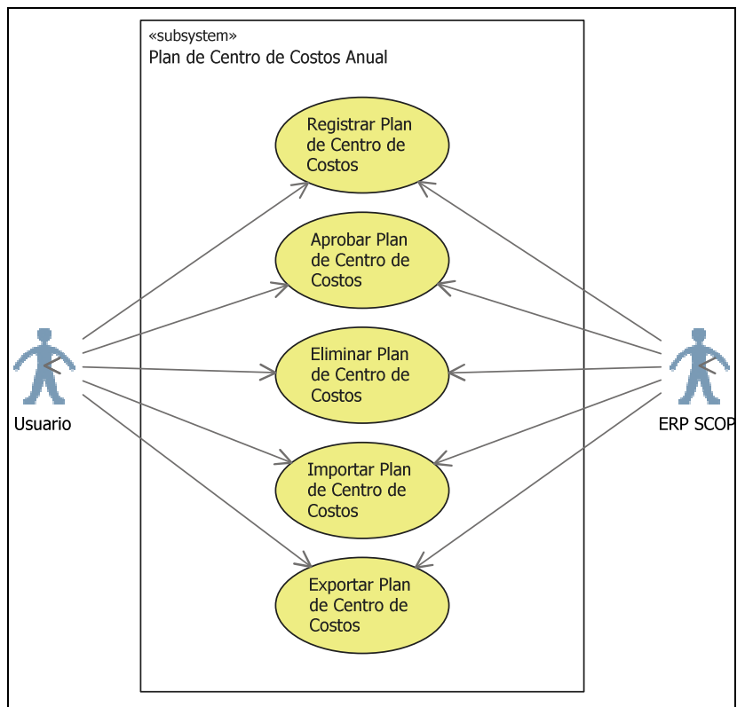
Figura 15. Diagrama de caso de uso Mantenimiento del Plan de Centros de Costos por Período Contable Anual
