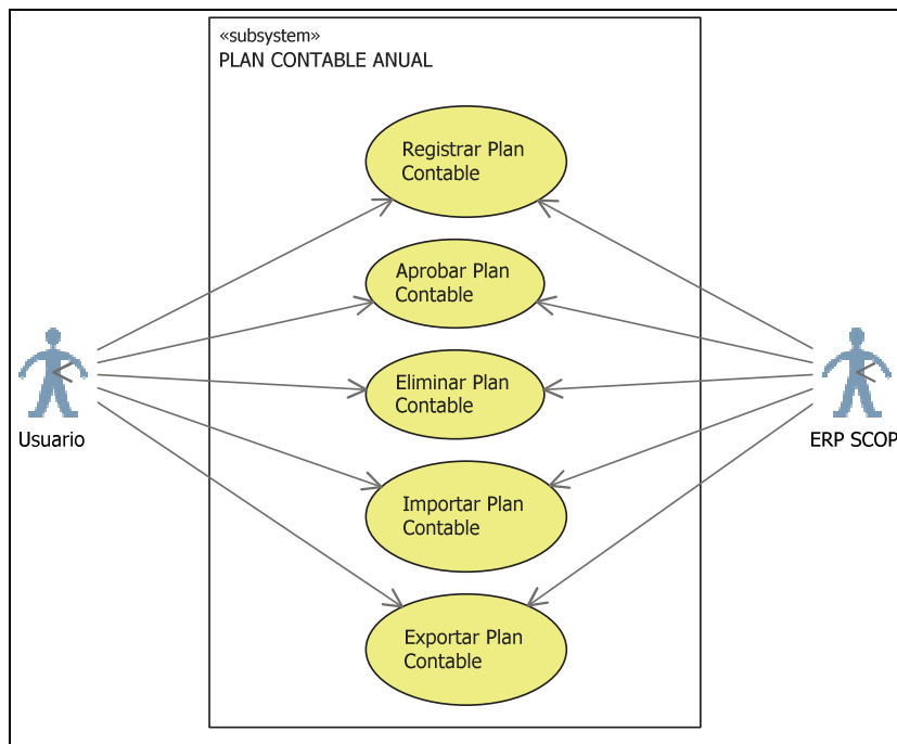
Figura 13. Diagrama de caso de uso Mantenimiento del Plan de Cuentas por Período Contable Anual
