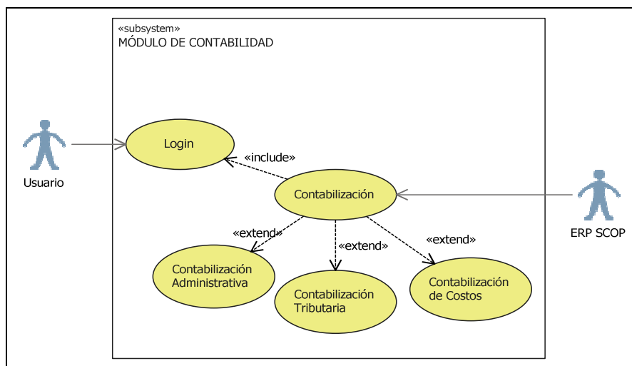
Figura 3. Diagrama de casos esenciales de uso
