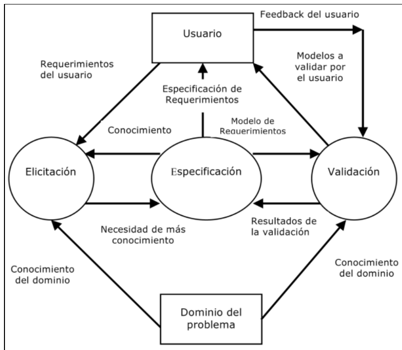
Figura 1. Procesos de ingeniería de requerimientos
