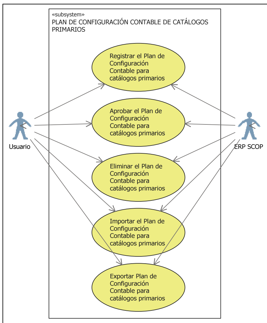
Figura 20. Diagrama de caso de uso Mantenimiento de los Planes de Configuración Contable Primaria
