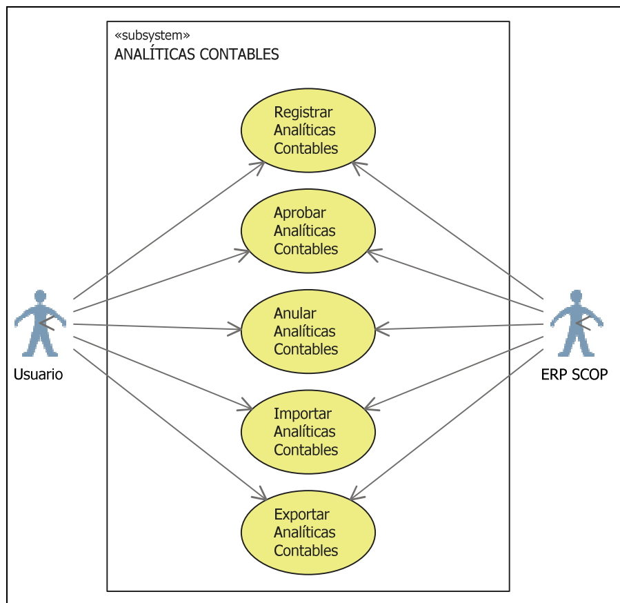
Figura 19. Diagrama de caso de uso Mantenimiento de las Analíticas Contables
