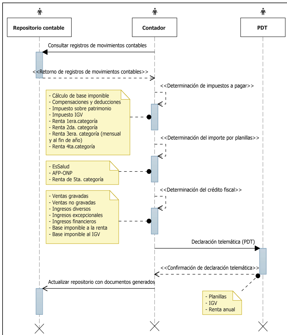
Figura 6. Diagrama de secuencia Contabilización Tributaria
